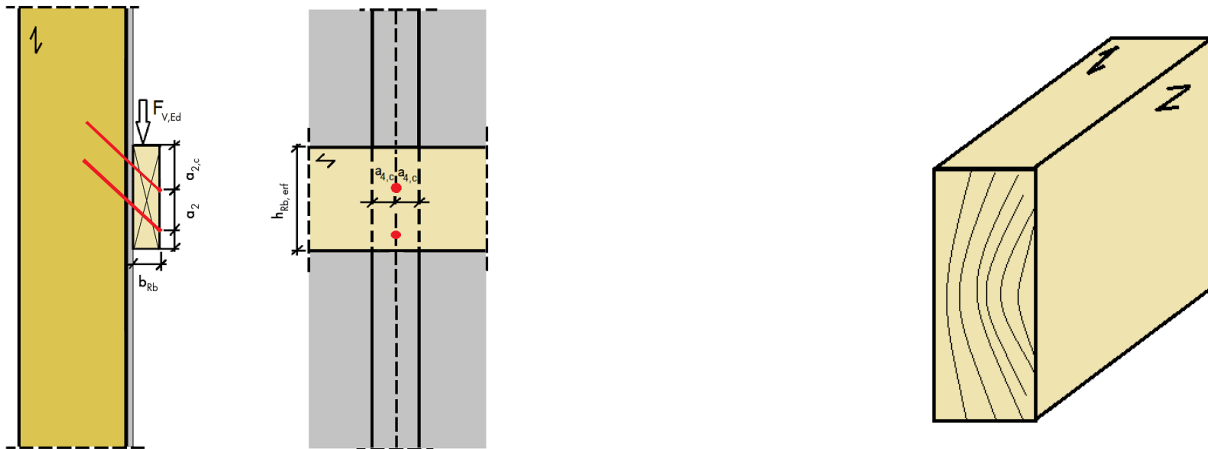
Charakteristische Tragfähigkeiten in kN von ASSY plus VG Vollgewindeschrauben (45°) Senk- /Zylinderkopfschrauben in Nadelholz C24, Nutzungsklasse 1 und 2
